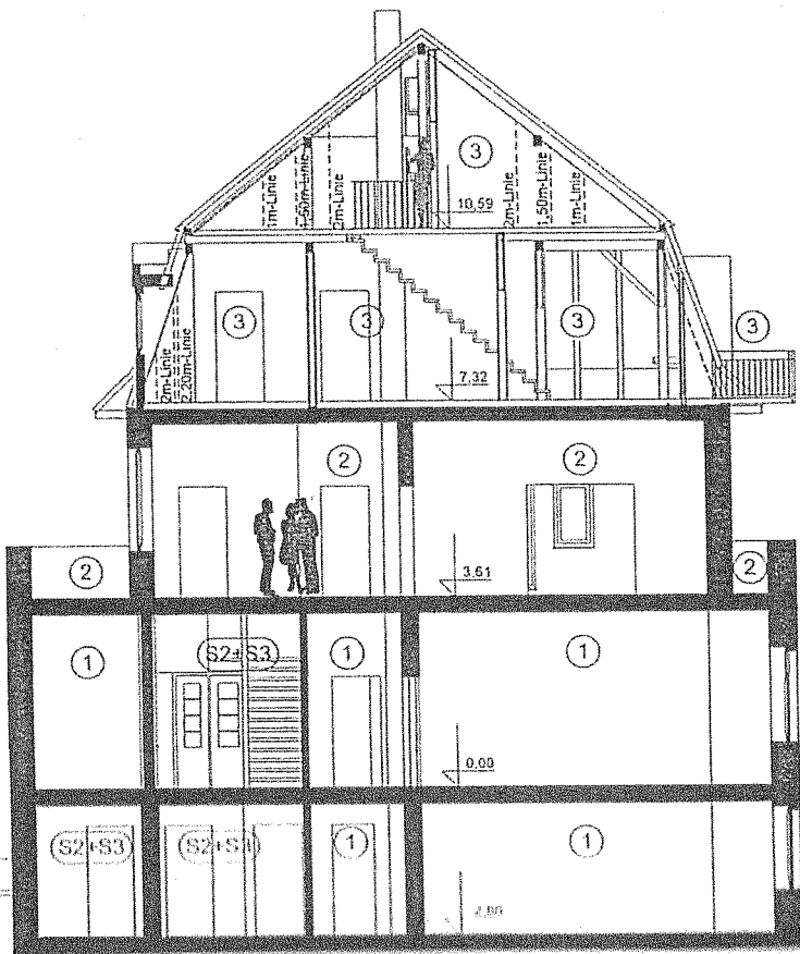
Schnitt 1-1 - Wohnung 3
