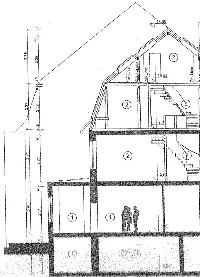
Schnitt 2-2 - Wohnung 3
